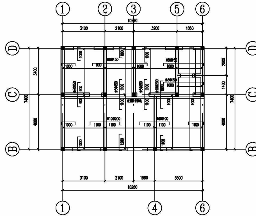
坡屋面配筋图
