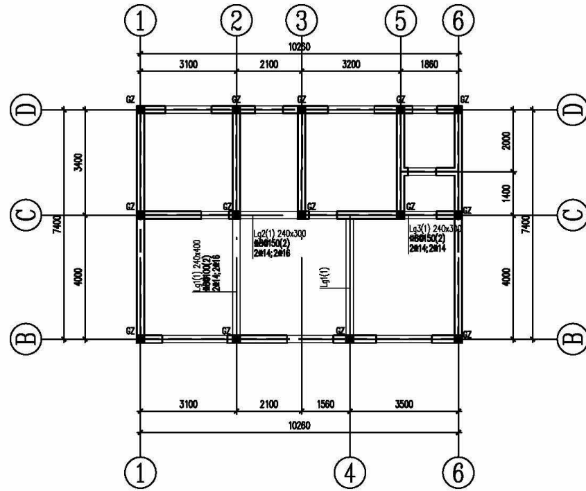
坡屋面结构平面布置图
