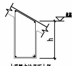
水平梁交坡屋面大样
